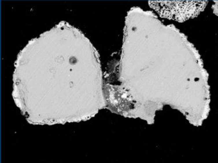
Elektronimikroskooppi BE-kuva
