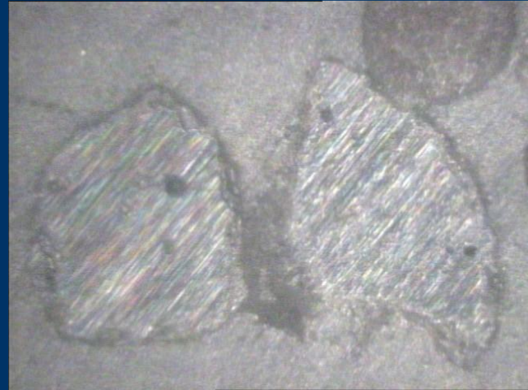
Valomikroskooppi
